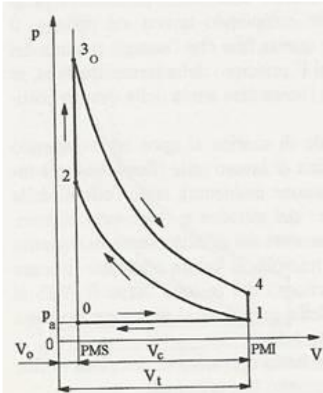
fig. 9.3 - Ciclo Otto
