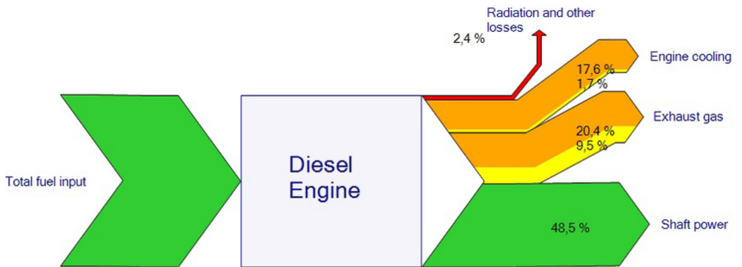
DIAGRAMMA FIUME – PERDITE/RENDIMENTI MCI DIESEL
