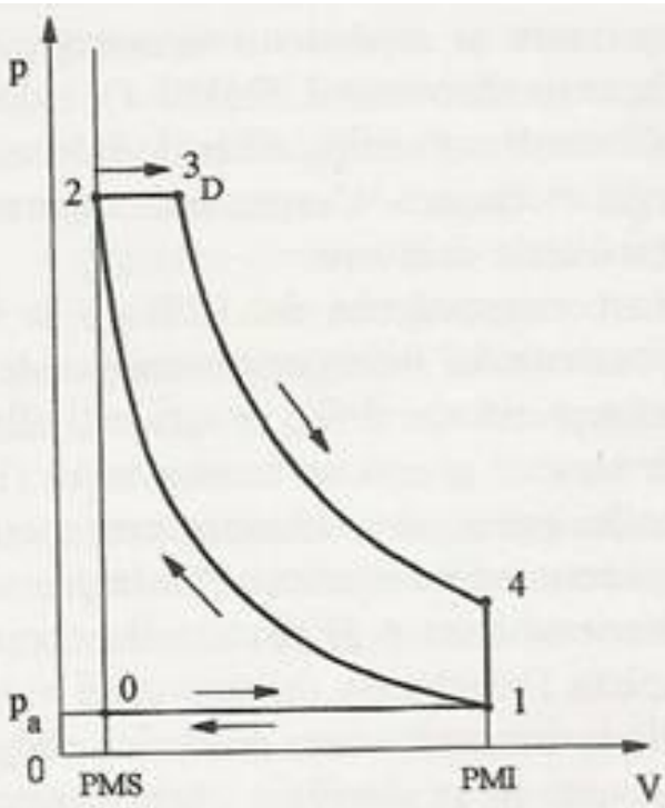
fig. 9.4 - Ciclo Diesel
